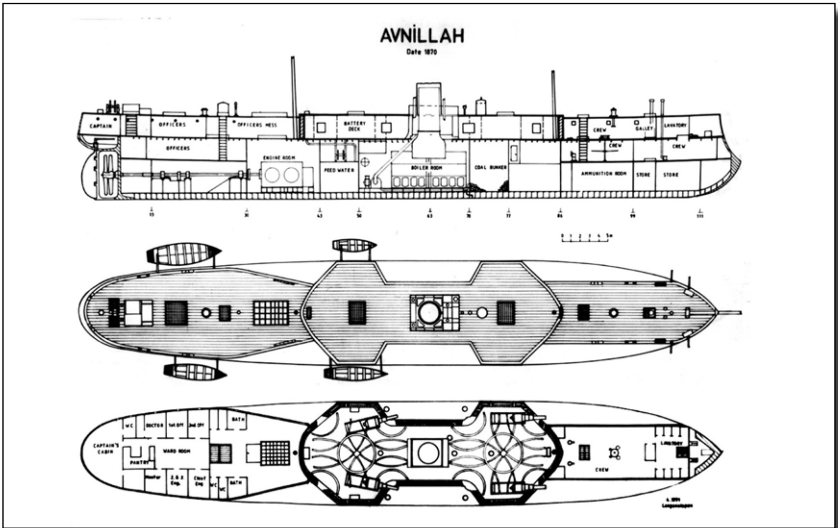
Avnillah korvetinin planı.
